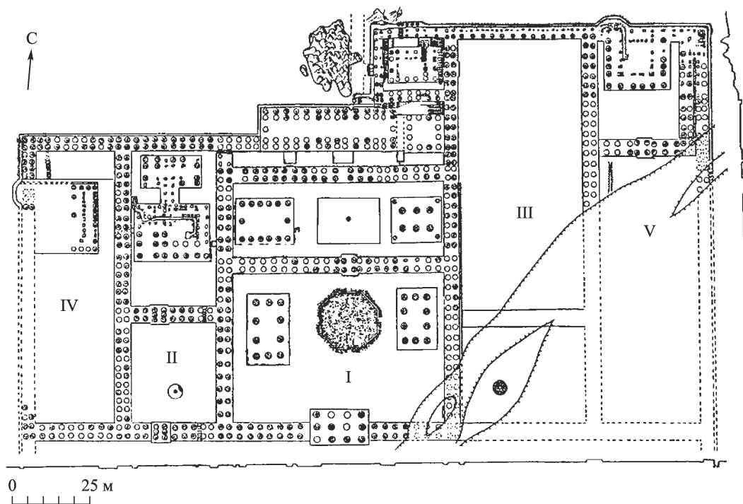
Рис. 1. План храмового комплекса Чоннынса (по: [Чо Хонгю, 2019, с. 118]).
